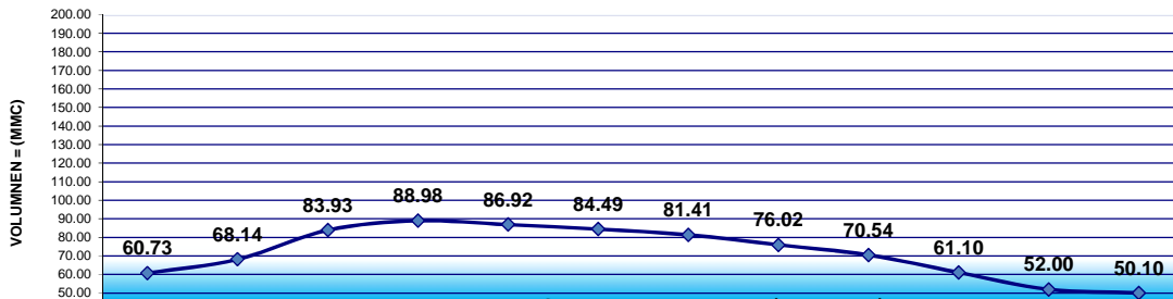
SALDO VOLUMEN EMBALSE PASTO GRANDE AÑO 2017
