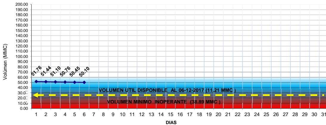
VARIACION DE VOLUMEN EMBALSE PASTO GRANDE DICIEMBRE 2017
